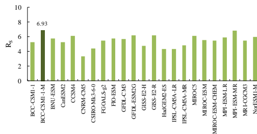
(d) Minimum temperature
